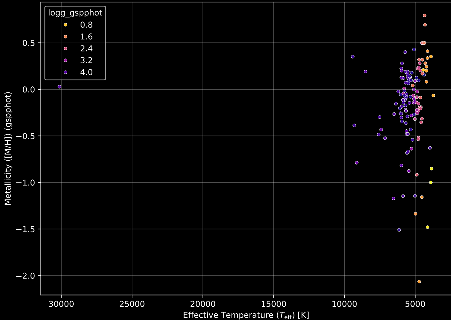
APOGEE DR17 Field: [278-31-O_TESS] Stellar Population Parameters (n= 131)
